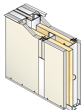
Exemple de cloison séparative
