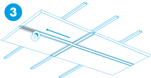
Collage de la bande sur les joints longitudinaux
