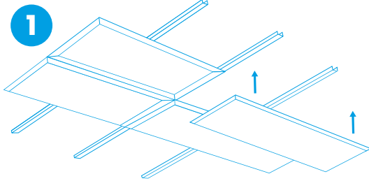
Possibilité d'aligner les joints transversaux
