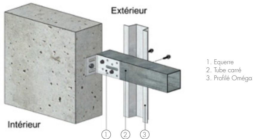
PRINCIPE DE FIXATION PAREMENT GLASAL DÉTAIL TUBE CARRÉ
