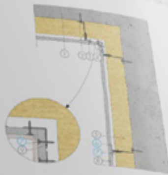
DISPOSITION DE VISE EN CORNER VISEE EN BOUTON SUR CORNER EN ALU
