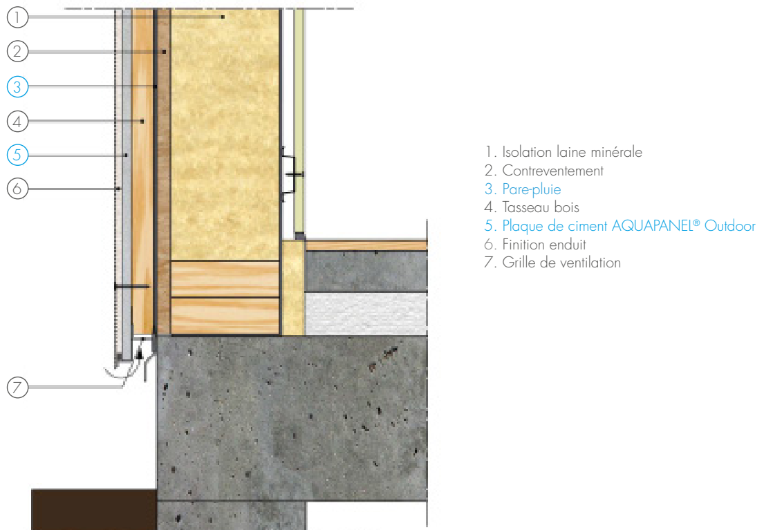
COUPE VERTICALE - PIED DE BARDAGE - OSSATURE BOIS SUR COB
