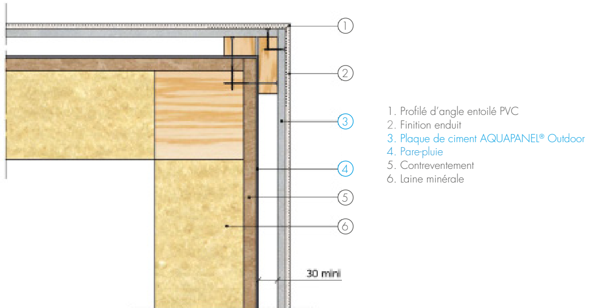
FIG 13 COUPE HORIZONTALE - ANGLE SORTANT - OSSATURE BOIS SUR SUPPORT COB
