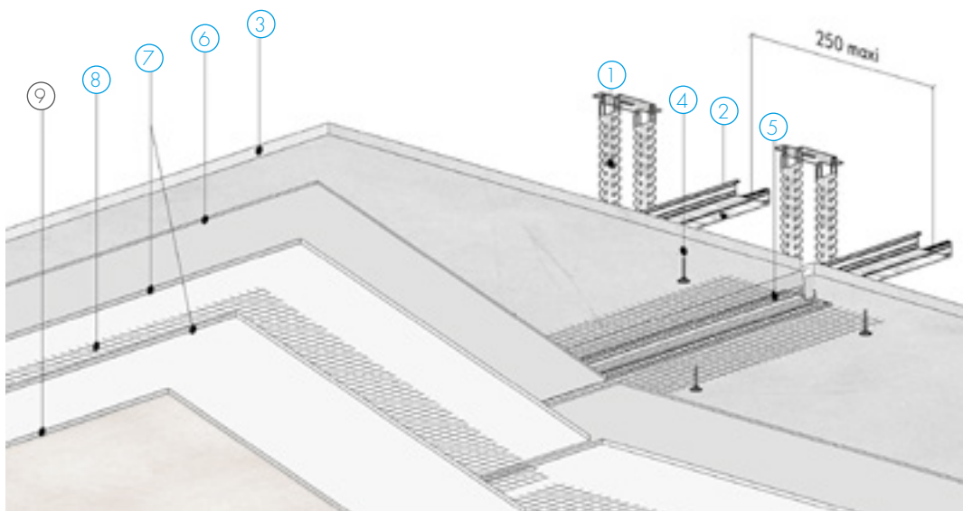
PRINCIPE DE MISE EN ŒUVRE DU PLAFOND AQUAPANEL® OUTDOOR
