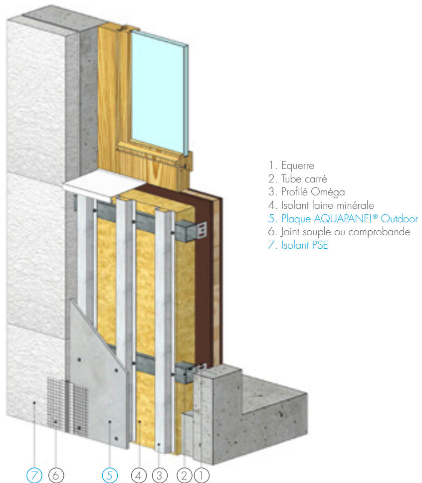
PRINCIPE DE FIXATION PAREMENT GLASAL
