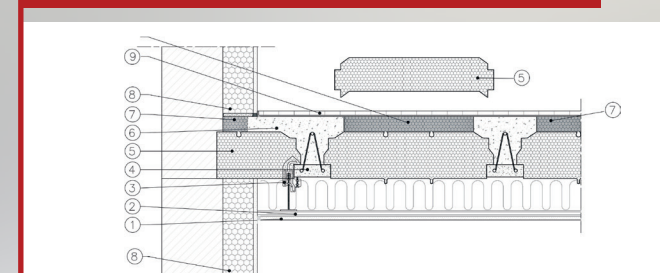
Entrevois isolant Knauf Treillis Therm G ou Knauf Treillis Therm coffrant avec Rupteur Knauf Stop Therm ULTRA
