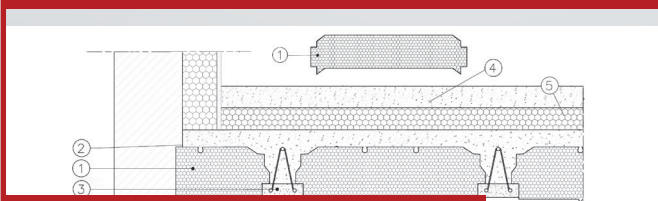
Mise en Oeuvre Solution Duo en Plancher Bas Knauf Treillis Therm G ou Knauf Treillis Therm Coffrant
