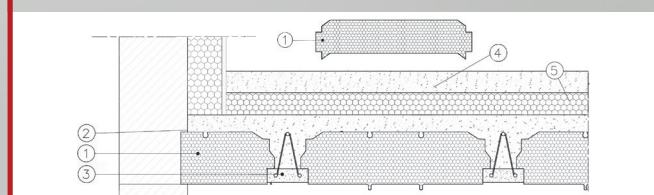
Mise en Oeuvre Solution Duo en Plancher Haut de sous-sol Knauf Treillis Therm G
