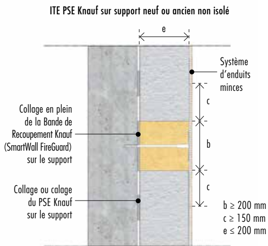
6 Coupe verticale sur la Bande de Recouvrement Knauf (SmartWall FireGuard) en partie courante
