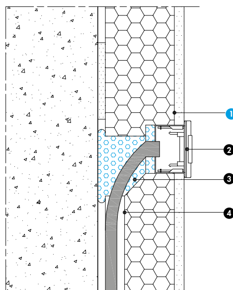
Fig. 4c : Étanchéité à l'air et des boîtiers électriques
