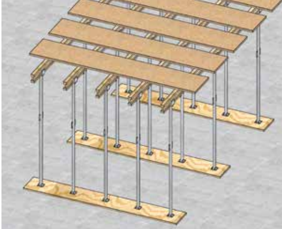
Fig. 1 : Pose et mise à niveau des planches ou bastinges
