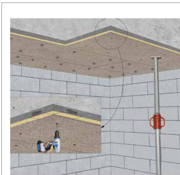
Fig. 13 : Fixation mécanique directe
