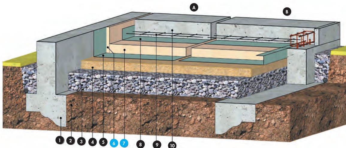
Fig. 1 : Dallage solidarisé/désolidarisé
