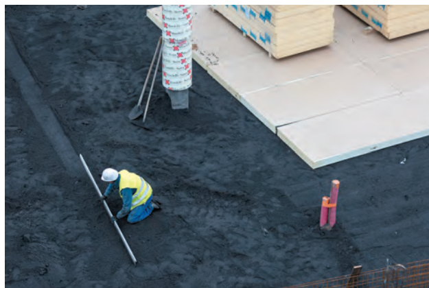
Couche de forme compactée et aplaniée, prête à recevoir les panneaux Knauf Thane Dallage
