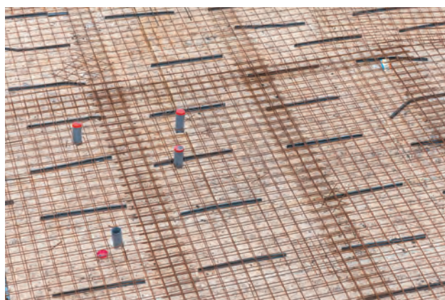
Double nappe de treillis d'armature de la dalle béton
