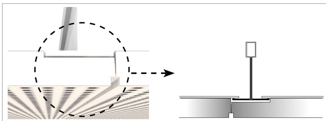
Dalle de plafond démontable Knauf Danoline - Unity 4 bord D+ (Contur)
