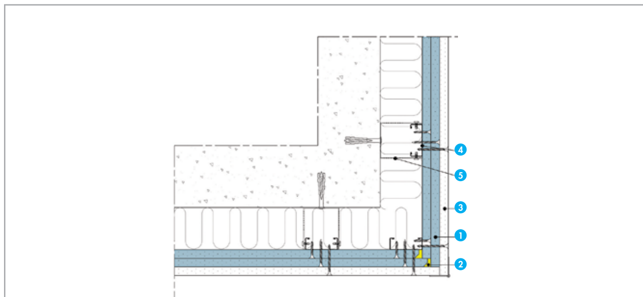
Fig. 15 : Angle sortant – F47
