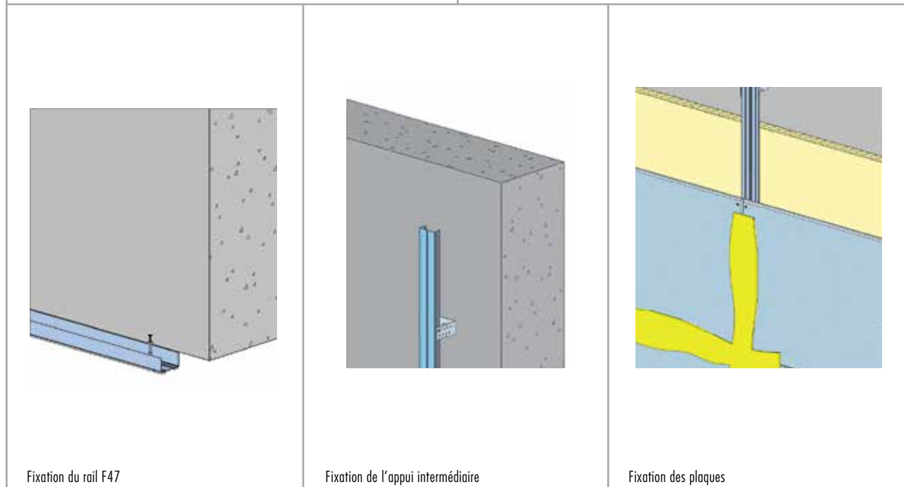
Fig. 11 : Contre-cloison Safeboard – F47
